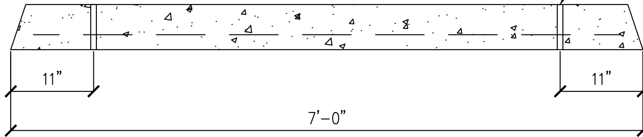
ELEVATION
